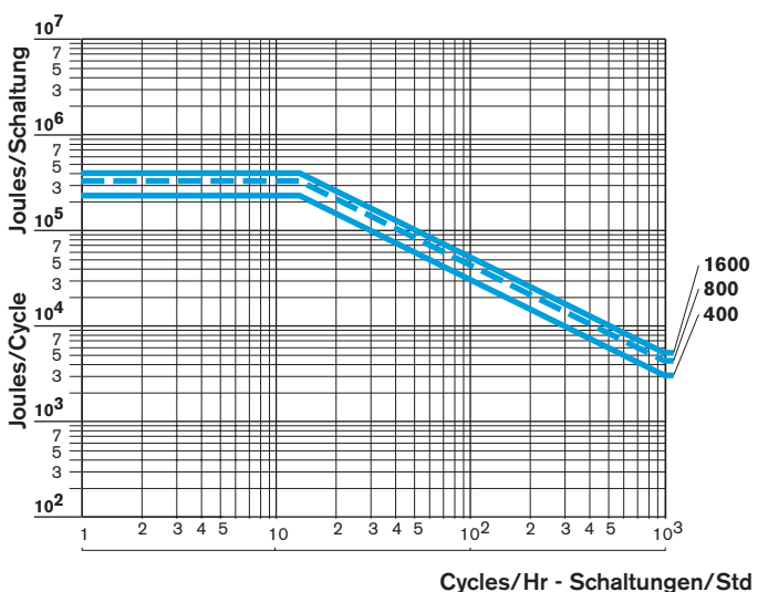
HEAT DISSIPATION / WÄRMEABFUHR VAR 02
